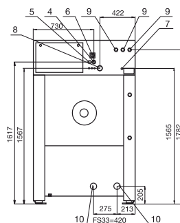
RÜCKANSICHT FS 33 40 55
