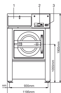
FRONTANSICHT FS 33 40 55
