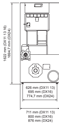
Seitenansicht DX 11 13 16 24 Elektrisch
