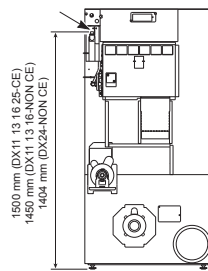
Rückansicht DX 11 13 16 24 Gas
