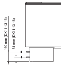
Obenseite DX 11 13 16 Dampf
