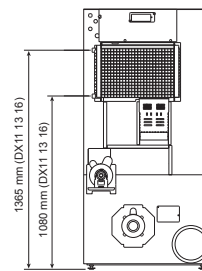
Rückansicht DX 11 13 16 Dampf
